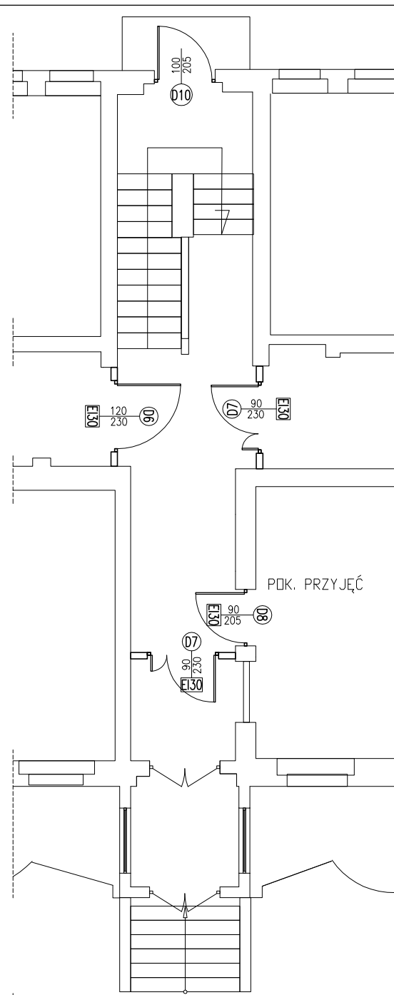
PARTER klatka schodowa 1:100
